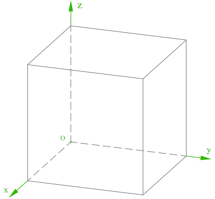
Oktaeder
