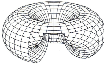
Aufgeschnittner Torus
